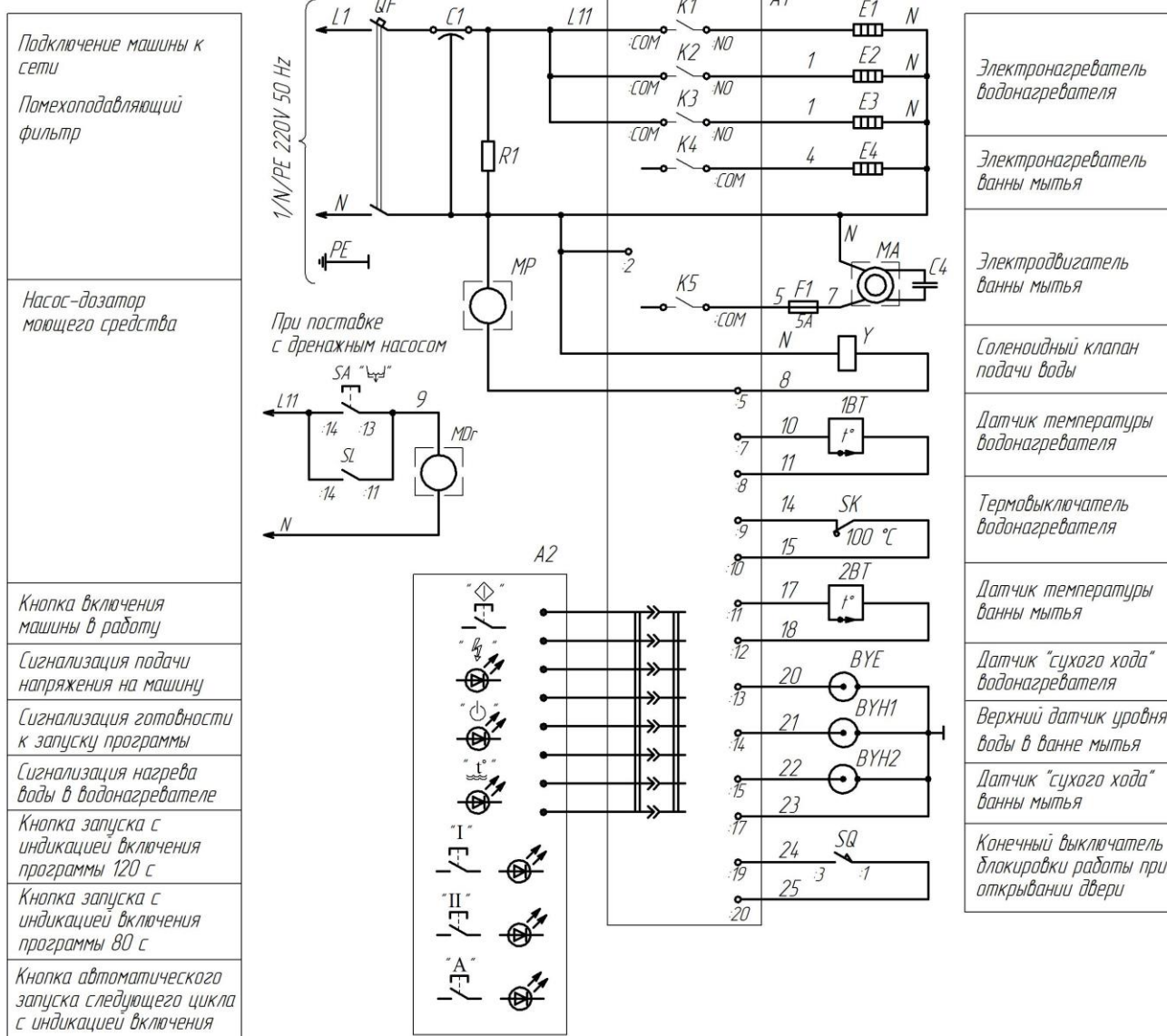
Схема машины МПФ-12-01-3 Остальное - см. схему МПФ-12-01
