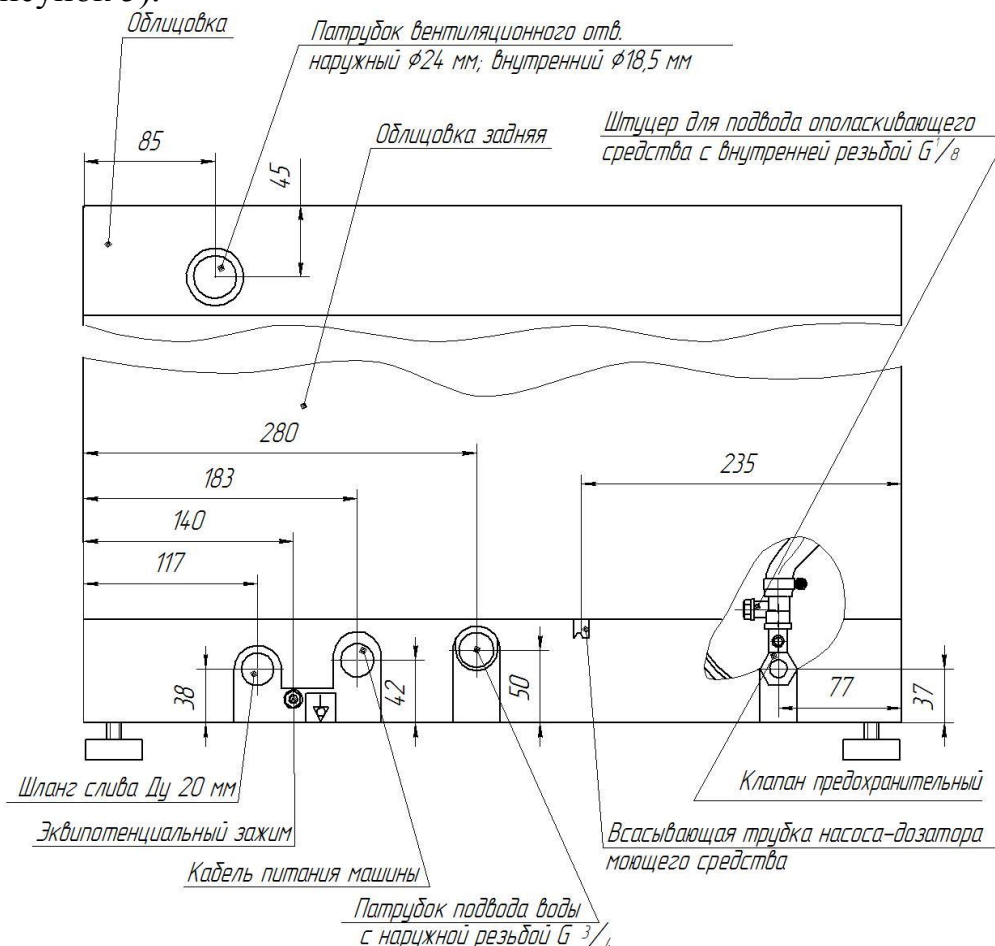
Рисунок 5 – Схема подвода коммуникаций к машине
