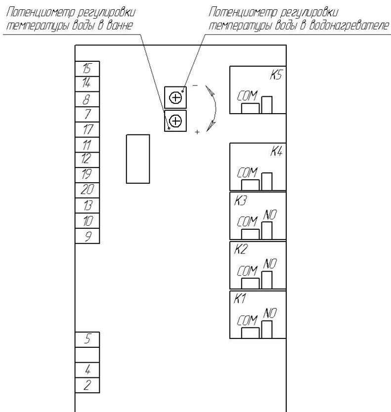
Рисунок 1 (лист 2 из 2) – Машина посудомоечная фронтальная МПФ-12-01
